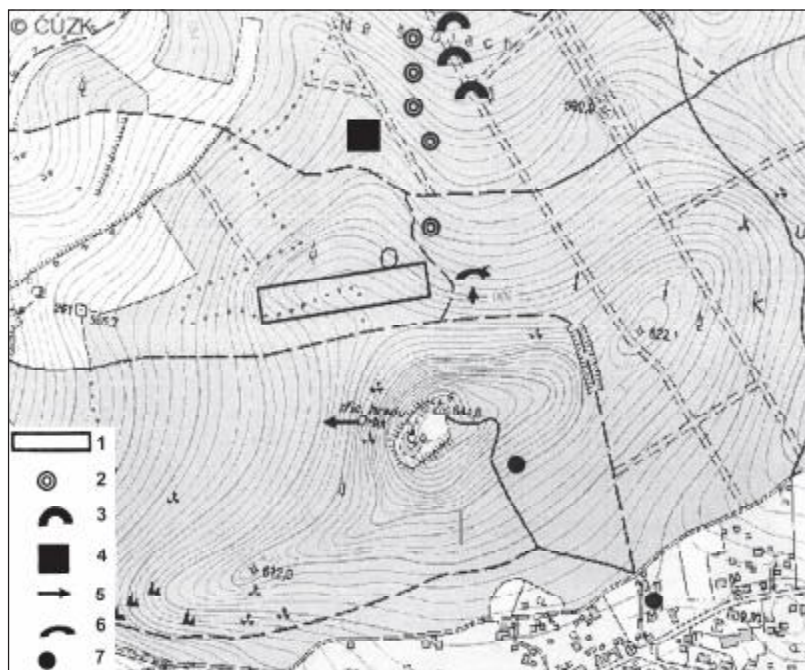
Obr. 1. Orlík u Humpolce. Celková situace výrobního areálu, hornických dobývek a hradu. 1 – hlavní dobývky na „Štůlách“; 2 – průzkumné pinky; 3 – rýžovnické kopečky-sejpy; 4 – rozpracované mlýnské kameny; 5 – výrony podzemní vody; 6 – hráz bývalého rybníka; 7 – hloubené studny. Podle J. Páši, upraveno
