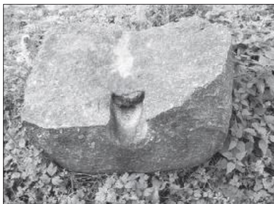
Obr. 10. Kašperské Hory. Mlýnský kámen rozlomený při vrtání dutým vrtákem. Obr. 2–7 a 10 foto J. Fröhlich
